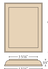
Rosette K-7318
