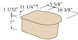
Starting End Cap K-8011 Specify LH or RH (RH Shown)
