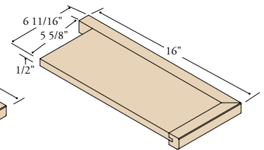
K-8071-2RE18 5-5/8" x 11-1/2" Specify LH or RH (RH Shown)
