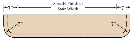
K-8060
