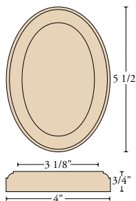
Rosette K-7337
