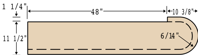
K-8010
